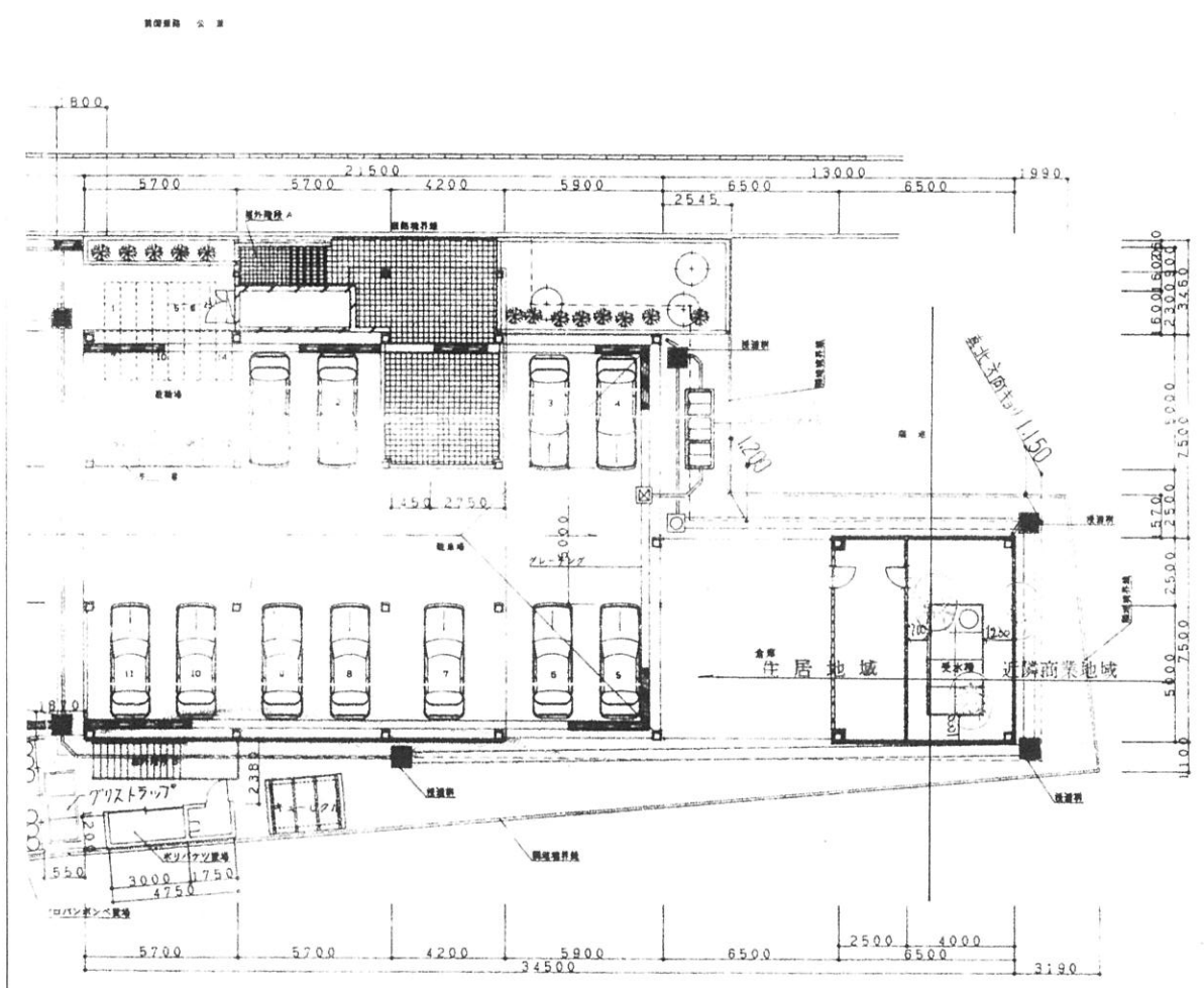
配置図 1階平面図 凡例 乙種防火戸
